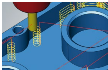
Restmaterialbearbeitung
