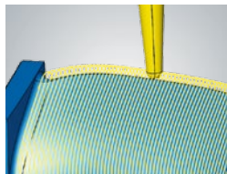
Punktkontakt-Schlichten
